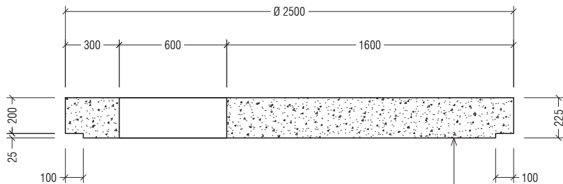
SECTION A-A (LID)
