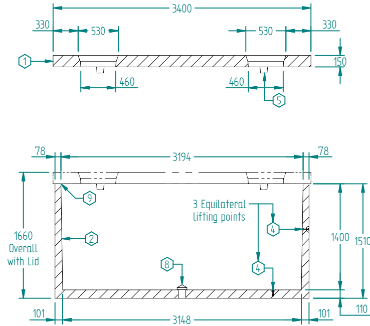
SECTION A-A 1:50
