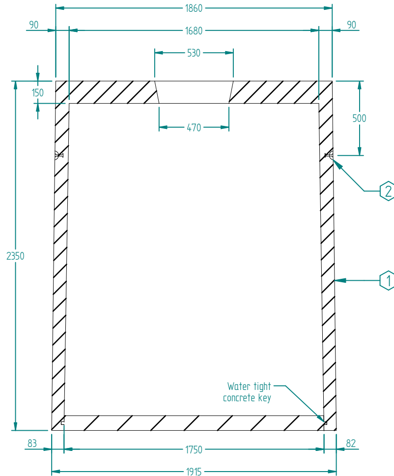
SECTION A-A 1:25
