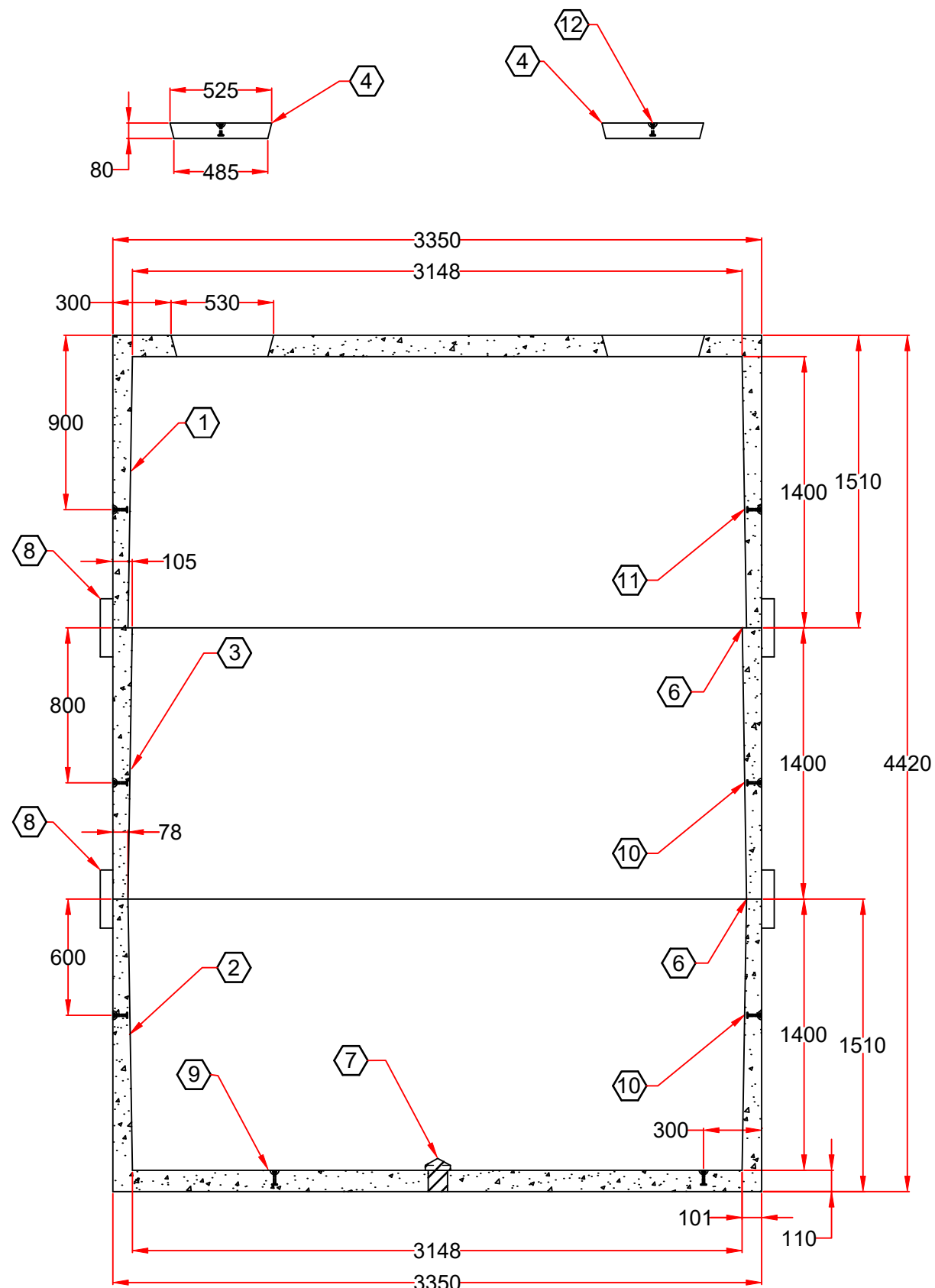
SECTION A-A
